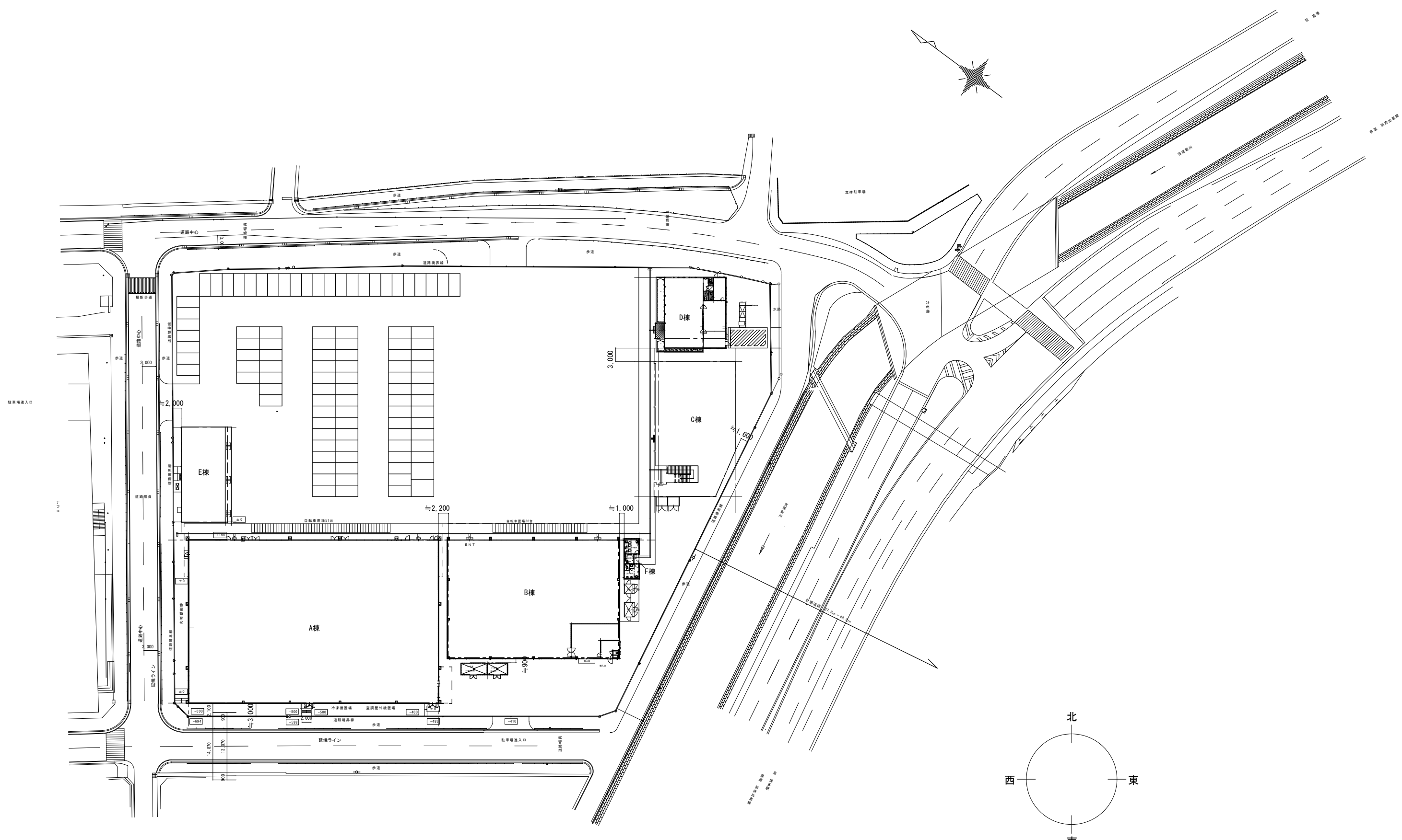
全体配置図 1/800
